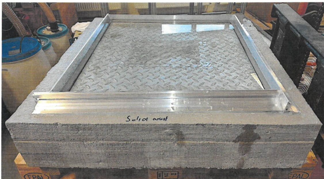
Obrázek 1: Zkouška vodotěsnosti - ACO Access Cover Solid ASSIST 600x600 B125
